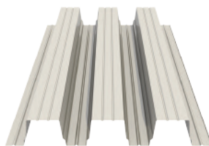
Профилированный лист H-75x750-A Толщина материала 0.65 - 1.0 мм
