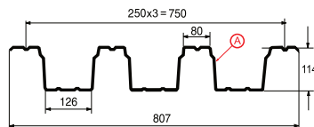
Профилированный лист H-114x750-A Толщина материала 0.7 - 1.0 мм
